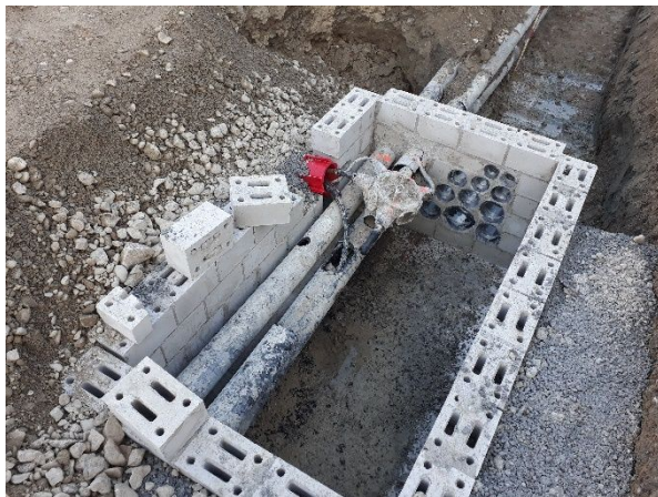
Abb. 1: Erstellung EW-Kabelschächte
