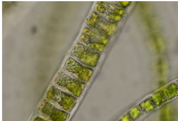
Ulothrix zonata , Fadenbreite: 30µm; Stelle: WAN_1
