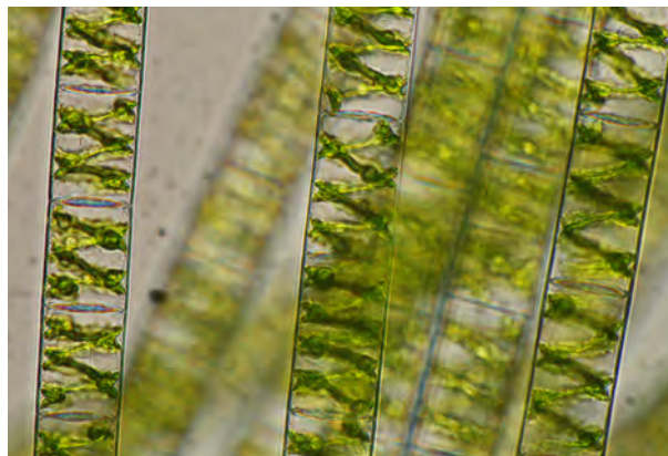
Spirogyra sp. , Fadenbreite: 40µm; Stelle: R-A_3
