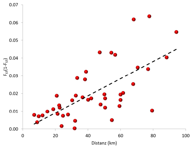
Abbildung 4-3. Mantel Korrelation zwischen der genetischen Distanz und der Gewässer-distanz aller natürlichen/wilden Populationen. Die Reuss_09 Population wurde bei dieser Analyse ausgenommen (siehe Text).
