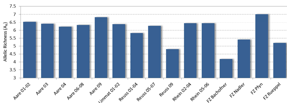
Abbildung 4-4. Anzahl Allele korrigiert für die Stichprobenzahl (Allelic Richness A_R ) für die verschiedenen Populationen.
