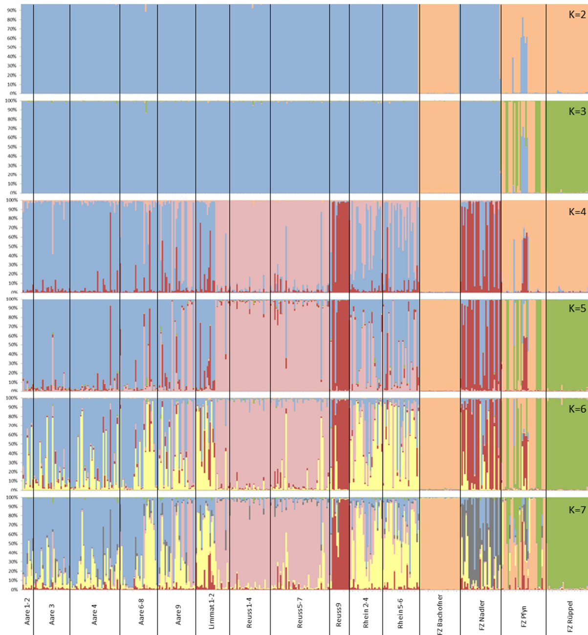
Abbildung 9-3. Resultate der Zuweisungsanalyse des Programms STRUCTURE für 2-7 hypothetische Populationen (K). Die verschiedenen genetischen Gruppen, die identifiziert werden, sind in unterschiedlichen Farben dargestellt. Jeder vertikale Balken entspricht einem Individuum.
