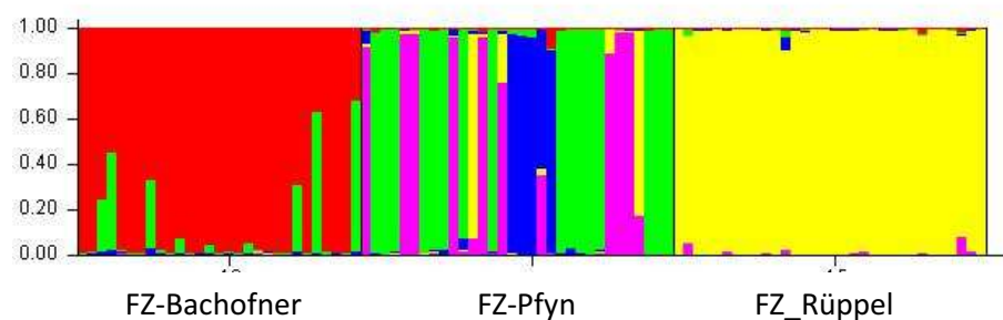
Abbildung 9-4. Resultate der Zuweisungsanalyse des Programms STRUCTURE für Die Zuchtpopulationen (K=5). Die verschiedenen genetischen Gruppen, die identifiziert werden, sind in unterschiedlichen Farben dargestellt. Jeder vertikale Balken entspricht einem Individuum.
