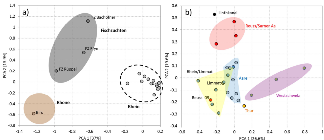
Abbildung 4-5. Hauptkomponentenanalyse der Äschenpopulationen der Schweiz. a) mit allen Populationen; b) ohne die vier Ausreisserpopulationen FZ_Bachofne, FZ_Pfyn, FZ_Rüppel und Birs.
