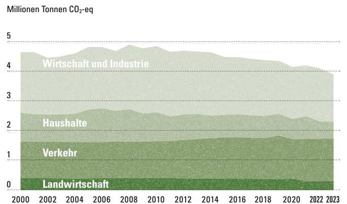
Treibhausgasemissionen nach Sektoren, Aargau
