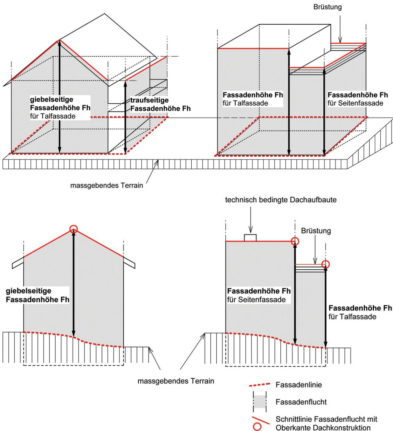
Figur 5.2 Fassadenhöhe
