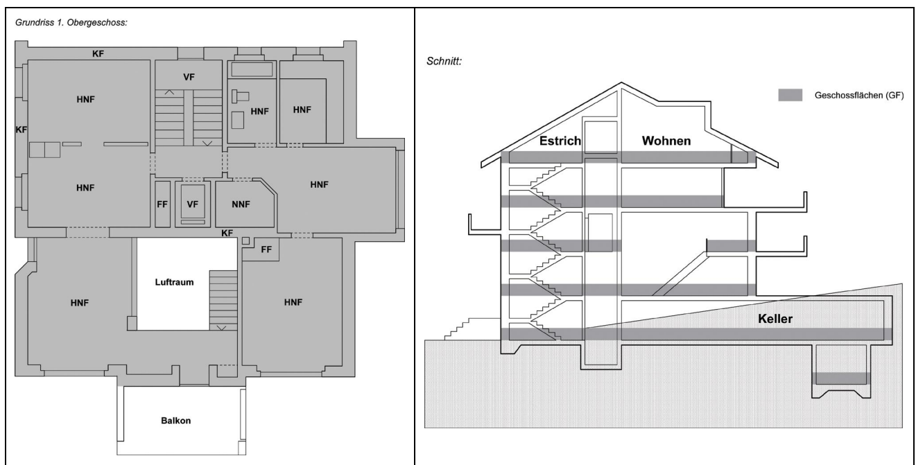
Figur 8.2 Geschossflächenziffer
