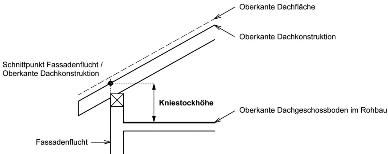
Figur 5.3 Kniestockhöhe
