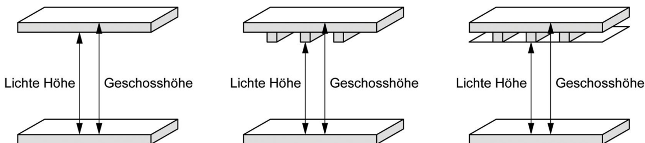
Figur 5.4 Lichte Höhe
