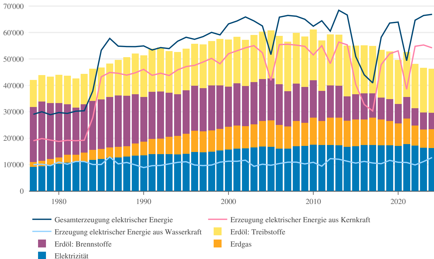
Abbildung 8.1: Energieverbrauch und Energieerzeugung im Kanton Aargau, in Terajoule, 1977–2024
