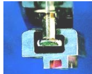
Pilzkopfzapfenverschluss bei Sicherheitsfenstern
